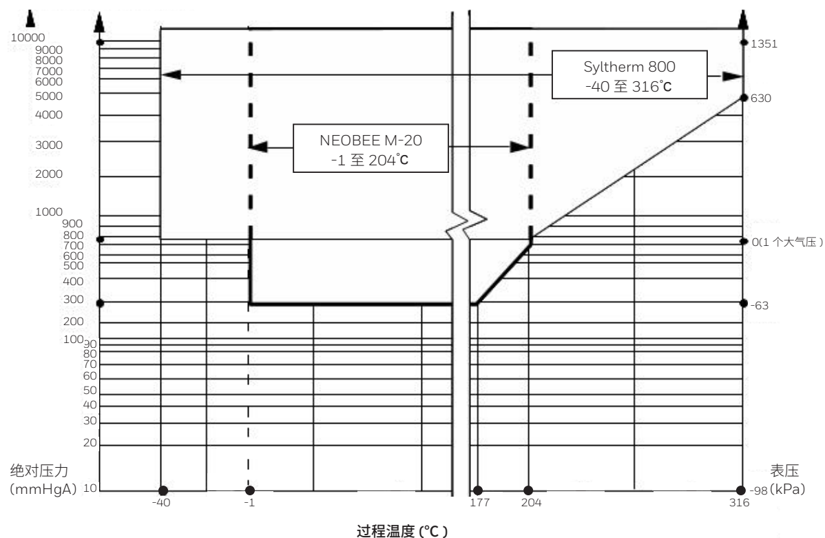
图 4 STR700 远传法兰常用充油操作压力与介质温度对应关系图
