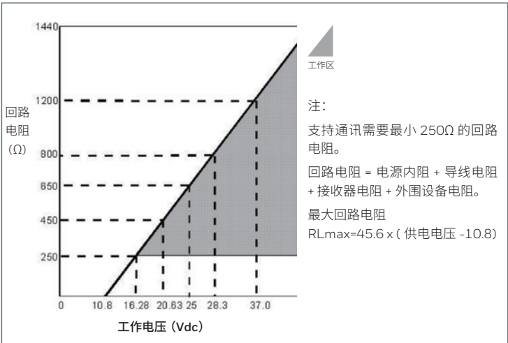
图 2 电源电压以及回路电阻图与计算
