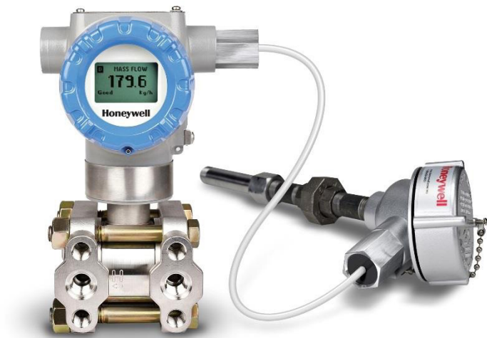
图 1 SMV800 多变量变送器
