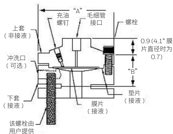
带下套的平法兰 (□)
