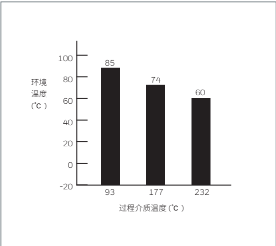
图 3 环境温度限制
