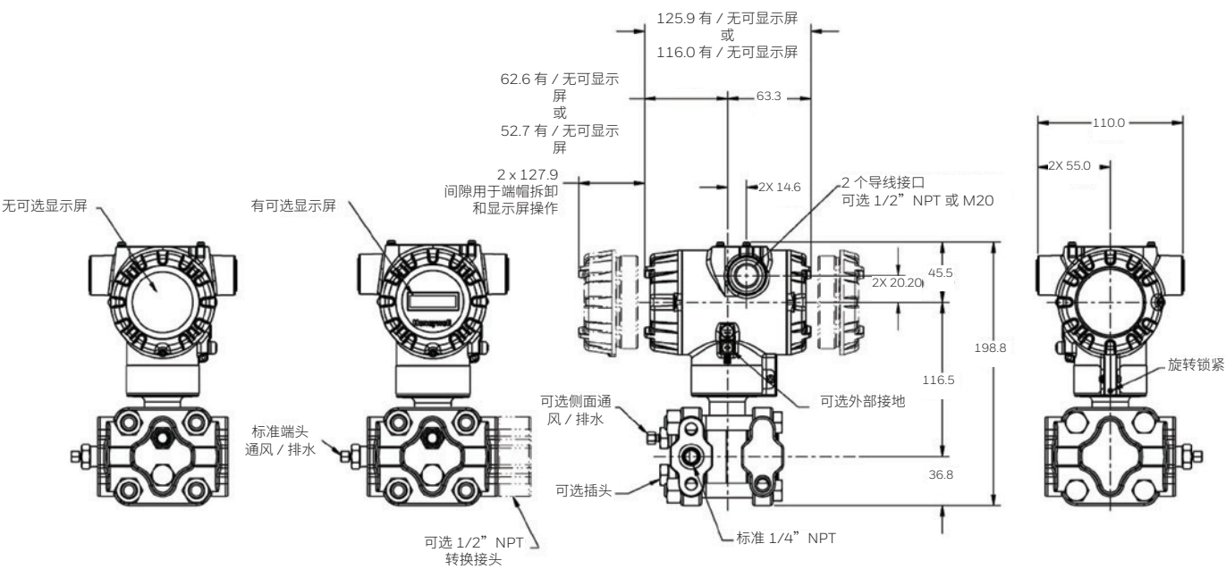
图 3 STD810, STD815, STD820, STD825, STD830 & STD870 的典型安装尺寸，供参考
