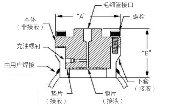
图 17 远传法兰尺寸 (4" 鞍形法兰)
