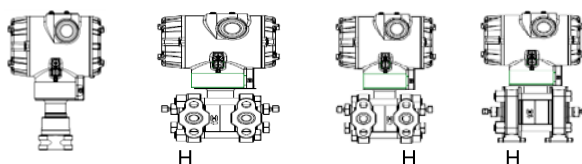
选项 1 标准 选项 2 高低压侧反向 选项 3 90° 旋转向下
