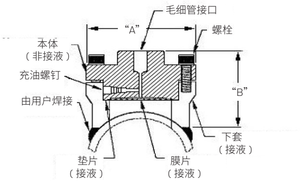
图 16 远传法兰尺寸 (3" 鞍形法兰)
