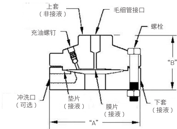
图 12 远传法兰尺寸 (螺纹式法兰)
